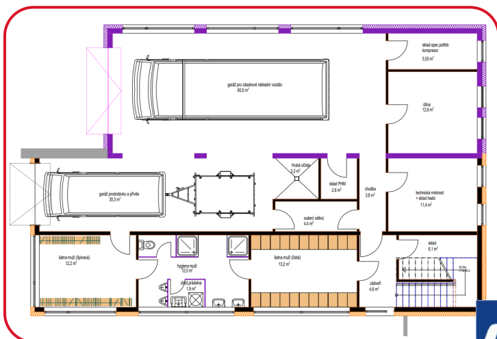
1. nadzemní podlaží
